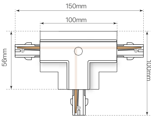
conexión T-IZQUIERDA-1
